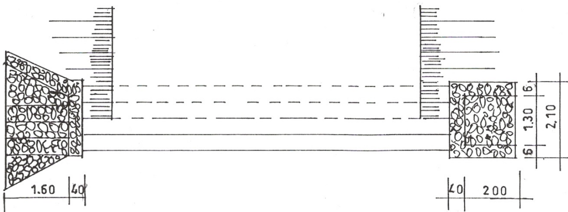
COUPE AA
