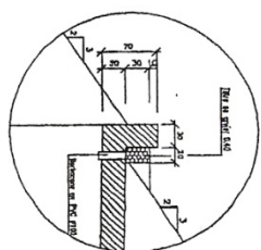
DETAIL "A" CON 1/23
