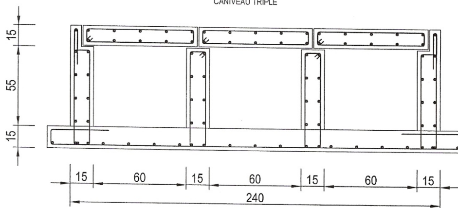
CANIVEAU TRIPLE
