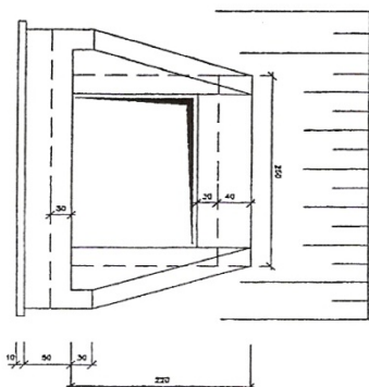
ELEVATION AVAL CON 1/23
