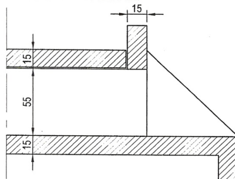
COUPE LONGITUDINALE
