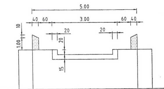
COUPE A-A
