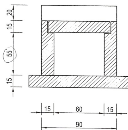
COUPE TRANSVERSALE
