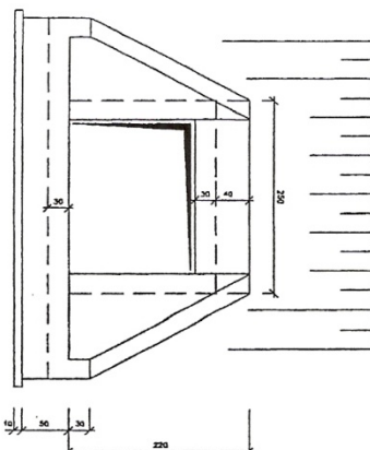
ELEVATION AMONT CON 1/23
